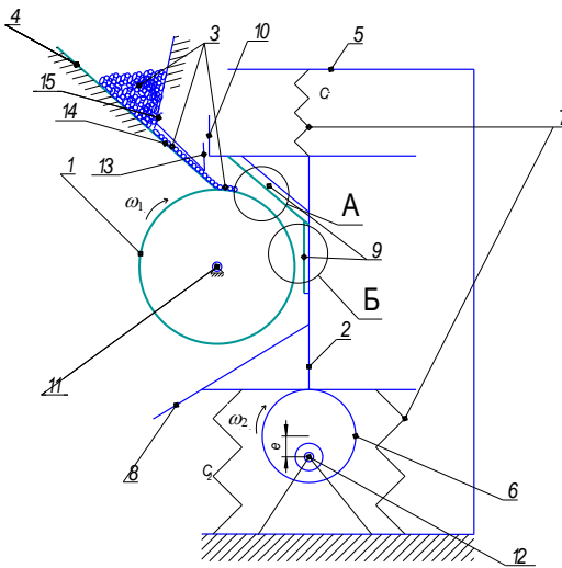
Рисунок 51 – Структурно-кинематическая схема одновальцево-декового измельчителя
