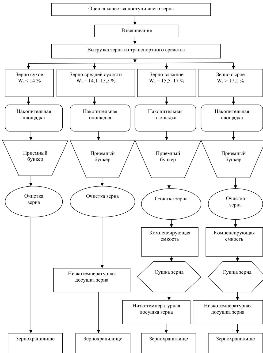
Рисунок 2. – Принципиальная схема разработанных поточных линий приема и послуборочной обработки зерна
