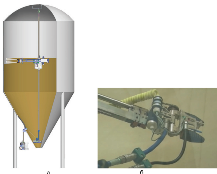
Рисунок 3. – Устройство внутренней очистки бункеров, производство компании Silo-RoBoFox (Германия): схема конструкции (а) и манипулятор с гидравлическими насадками (б)
