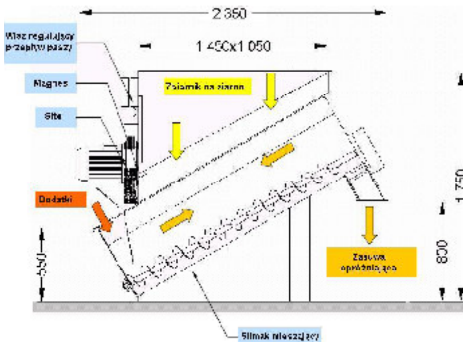
Rys. 2. Zestaw do rozdrabniania i mieszania paszy: 1 – włącz regulujący przepływ paszy, 2 – magnes, 3 – ruszt [materiały informacyjne firmy ELECTRA]
