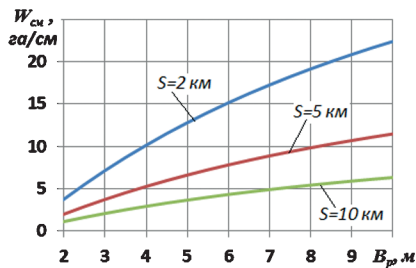
Рисунок 1. – Зависимость сменной производительности от ширины захвата машины для диапазона расстояний перевозки 2–10 км (доза внесения 40 м/га)
