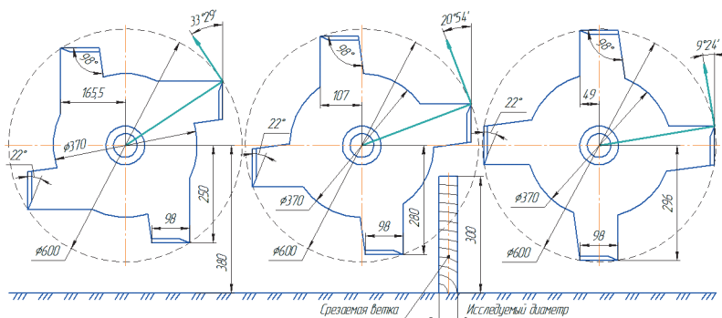
Рисунок 2. – Схема моделируемого опыта
