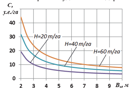
Рисунок 4. – Зависимость прямых удельных издержек от ширины захвата машины для диапазона доз внесения 20–60 м/га (расстояние перевозки 4 км)
