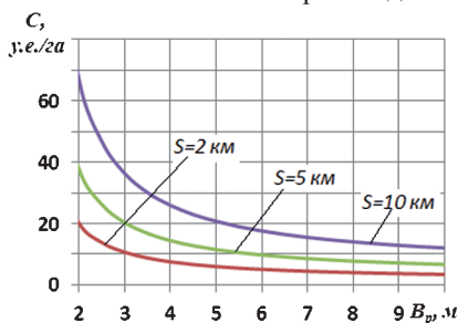
Рисунок 3. – Зависимость прямых удельных издержек от ширины захвата машины для диапазона расстояний перевозки 2–10 км (доза внесения 40 м/га)
