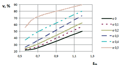
Рисунок 1. – Зависимость точности посева от коэффициента внутреннего трения семян при разных среднеквадратических отклонениях размеров семян
