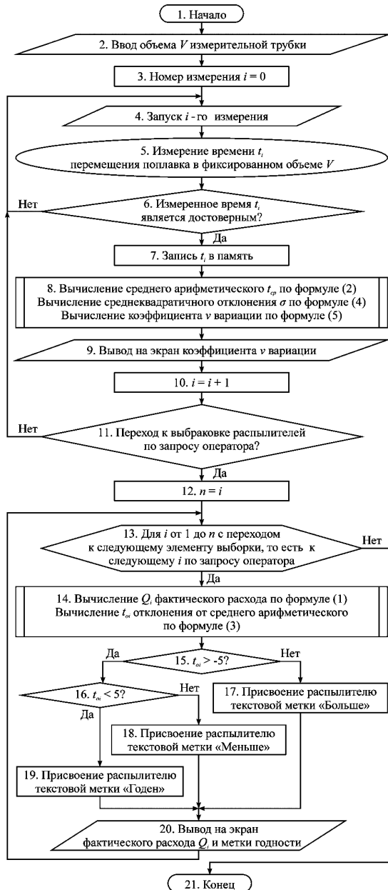
Рисунок 2. – Блок-схема алгоритма оценки качества работы опрыскивателей в полевых условиях
