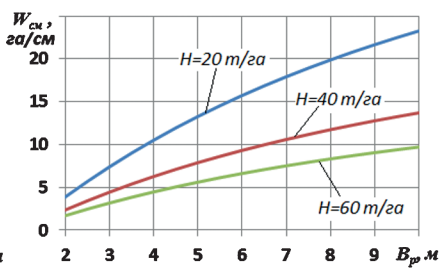
Рисунок 2. – Зависимость сменной производительности от ширины захвата машины для диапазона доз внесения 20–60 м/га (расстояние перевозки 4 км)
