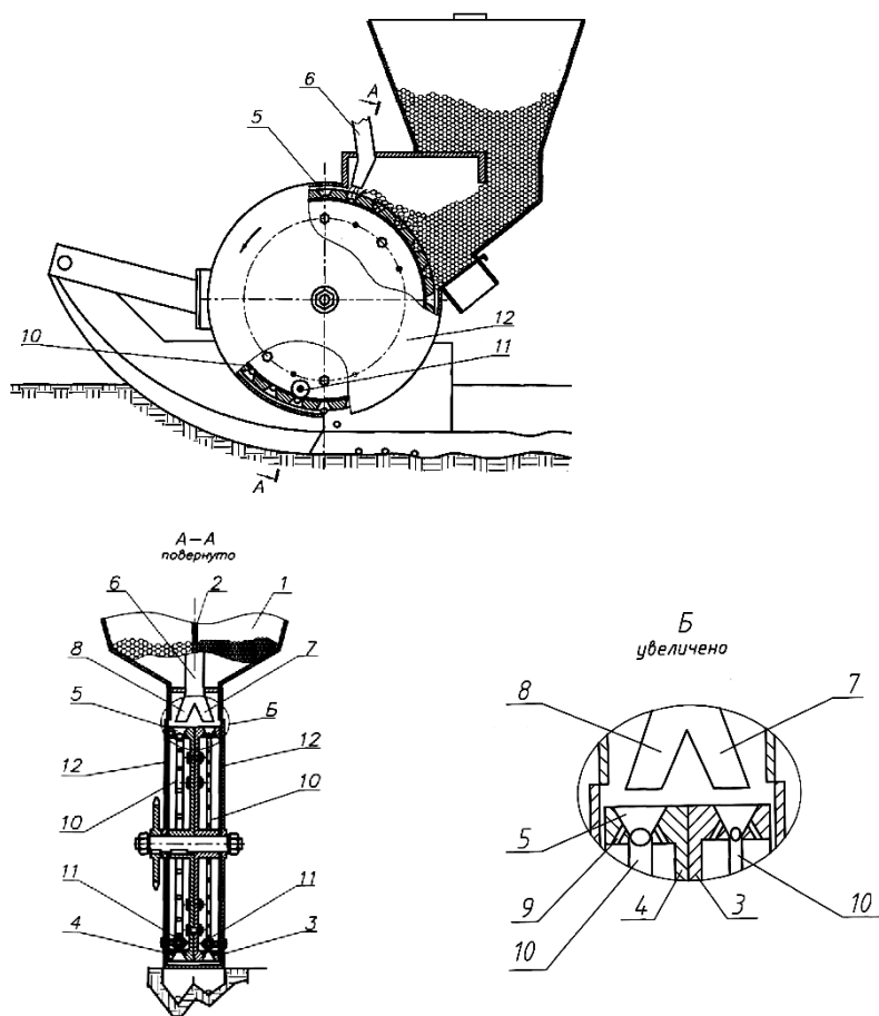
Рисунок 2. – Пневматический высеваящий аппарат
