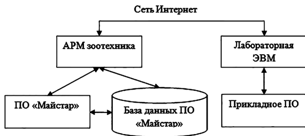
Рисунок 3. – Удаленный сбор экспериментальных данных о параметрах дойки с использованием глобальной сети Интернет
