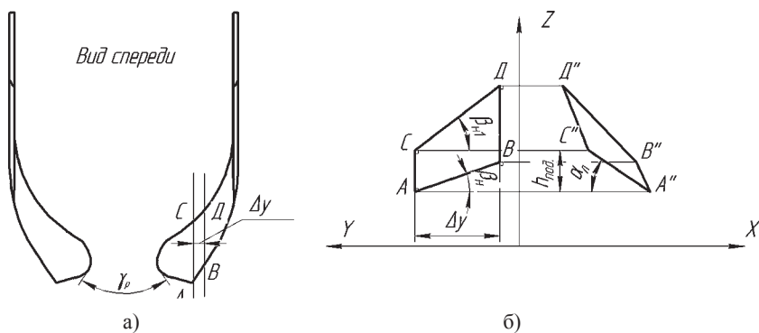
а) подкапывающий рабочий орган; б) проекция элементарного клина подкапывающего рабочего органа
