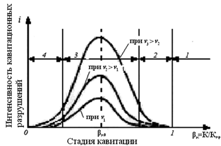
Рисунок 3. – Схематический график зависимости интенсивности кавитационных разрушений i от стадии кавитации \beta = K/K_{kp}
