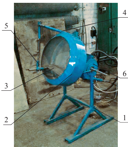
1 – станина; 2 – барабан; 3 – скатная доска; 4 – кронштейн; 5 – шарнир; 6 – механизм регулирования угла наклона барабана
