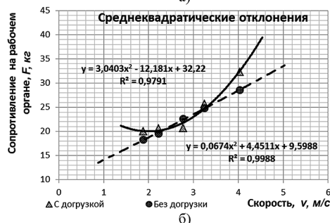
Рисунок 4. – Зависимости средних значений силы сопротивления на рабочем органе (а) и обобщенной координаты (б) от скорости орудия
